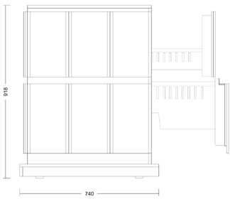
VUE LATÉRALE
