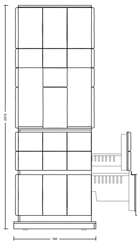
VUE LATÉRALE
